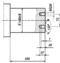
Wal silnika
